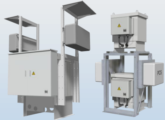
PPSC® NEW series 200kVA スマートタワーラック
